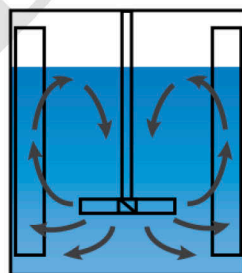
Hélice centrada con deflectores
