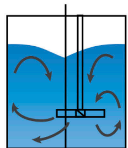
Hélice descentrada
