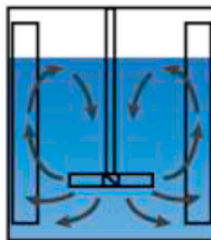
Hélice centrada con deflectores
